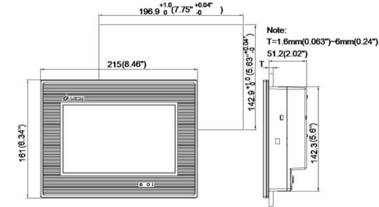
DOP-B07S(E)415 / DOP-B07PS415
