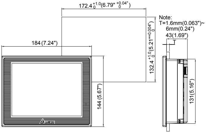
DOP-B07S(E)515 / DOP-B07PS515
